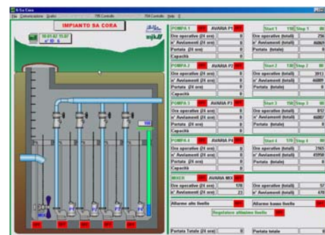
Da MJK-Link™: Stazione di sollevamento con 4 pompe e mixer
