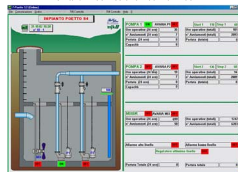
Da MJK-Link™: Stazione di sollevamento con 2 pompe e mixer
