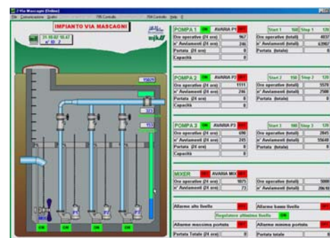
Da MJK-Link™: Stazione di sollevamento con 3 pompe e mixer
